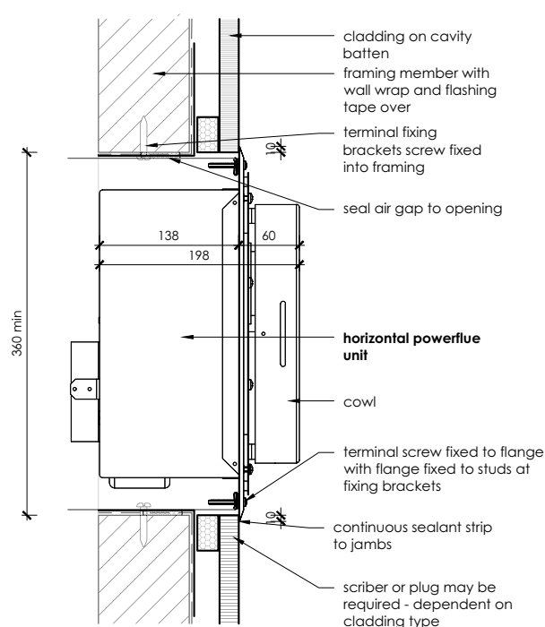
Jamb
