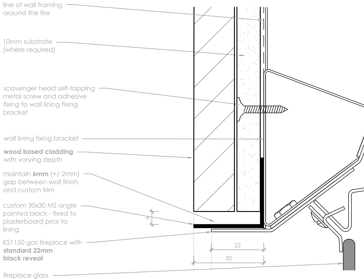
Custom L-Angle
